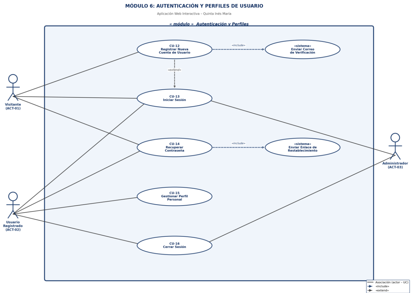
Figura: Diagrama CU – Módulo 6: Autenticación y Perfiles de Usuario
