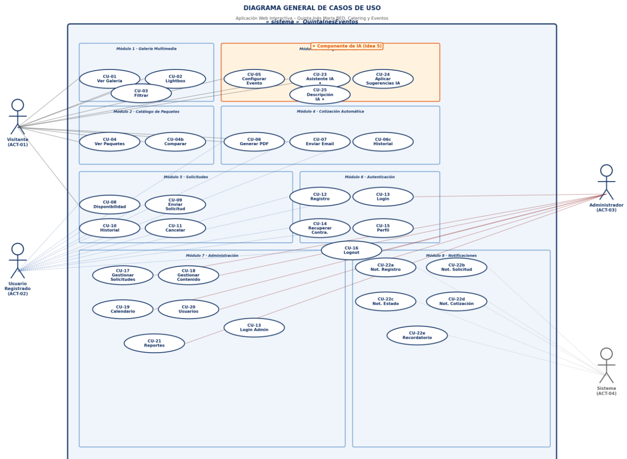
Figura: Diagrama General de Casos de Uso – QuintalinesEventos (incluye IA)
