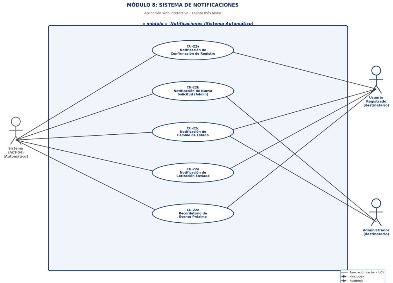
Figura: Diagrama CU – Módulo 8: Sistema de Notificaciones
