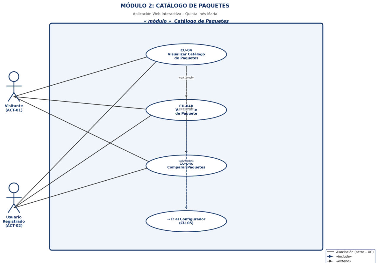
Figura: Diagrama CU – Módulo 2: Catálogo de Paquetes
