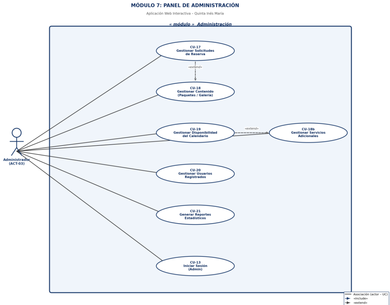
Figura: Diagrama CU – Módulo 7: Panel de Administración
