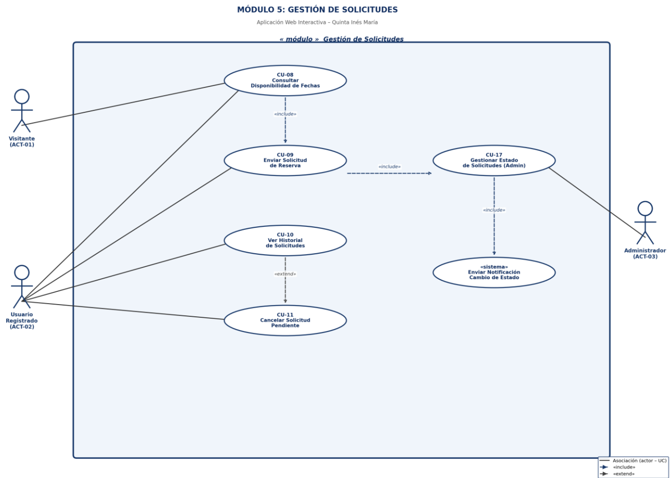
Figura: Diagrama CU – Módulo 5: Gestión de Solicitudes
