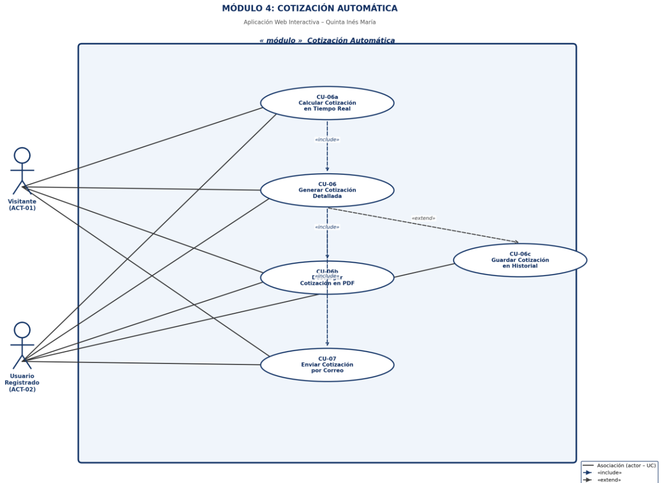
Figura: Diagrama CU – Módulo 4: Cotización Automática
